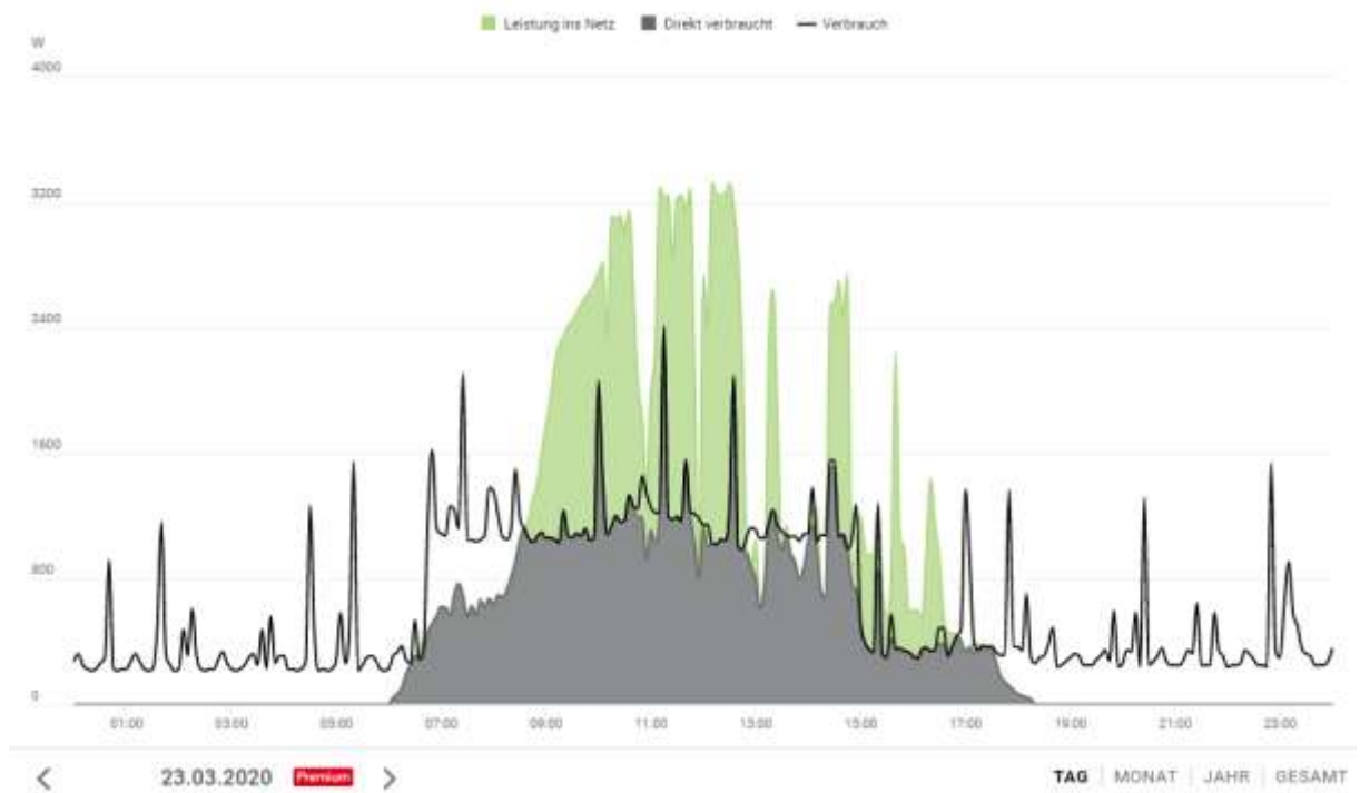
Typischer Tagesverlauf von Produktion und Verbrauch an einem wechselhaften Wochentag im März 2020
