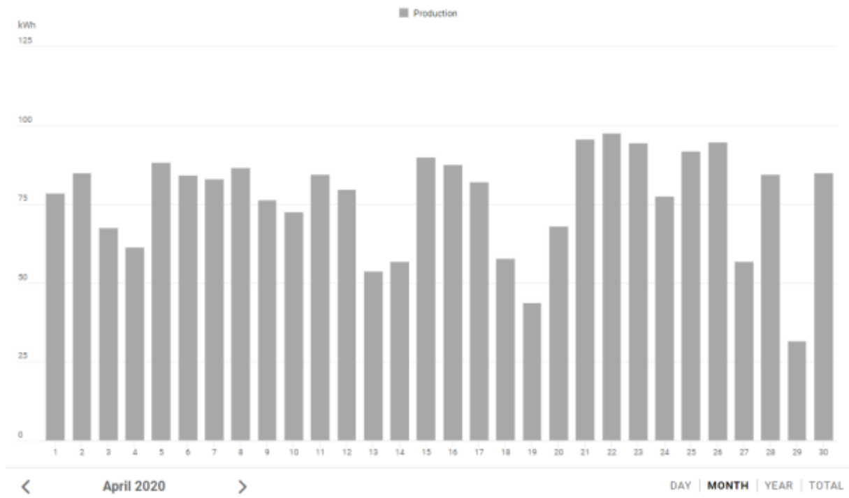
Produzierte Tagesenergie im April 2020 (Volksschule)
