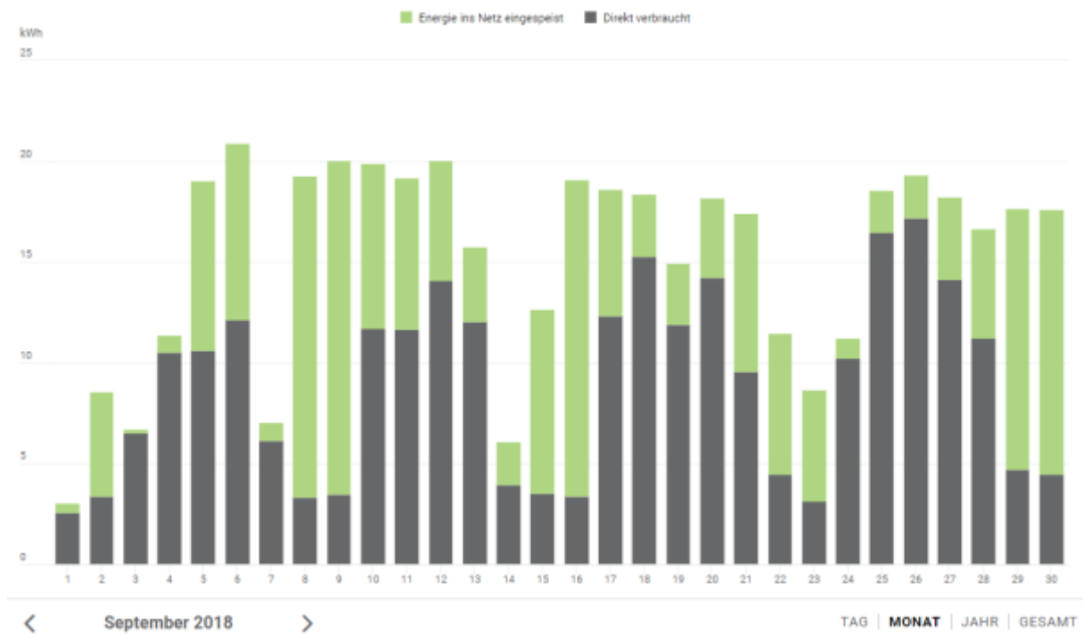
Produzierte Tagesenergie im September 2018 (weniger Verbrauch am Wochenende)
